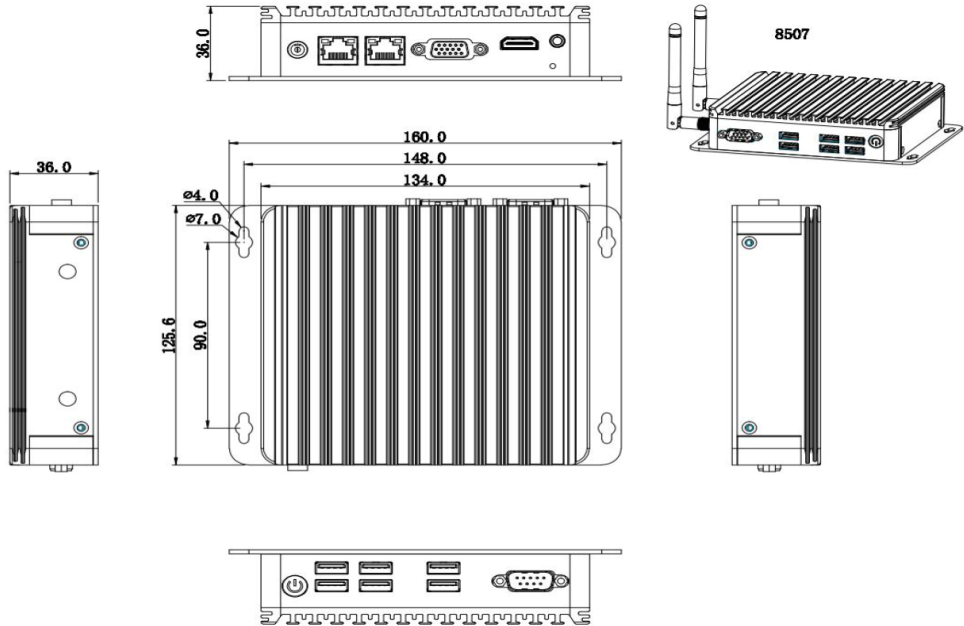
单位：mm
